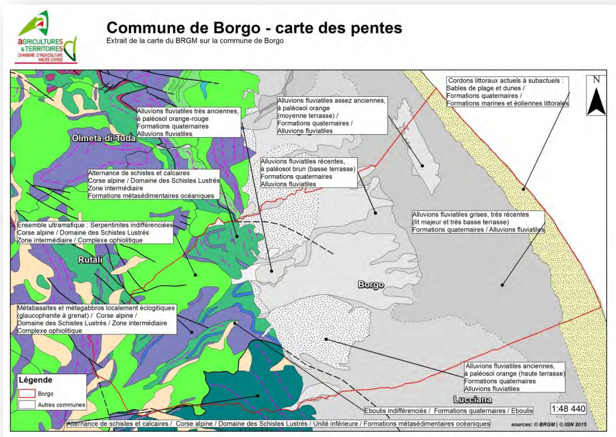
CARTE 7 : GEOLOGIE DE LA COMMUNE DE BORGO (SOURCE : BRGM, CREATION CARTE : CA 2B)
